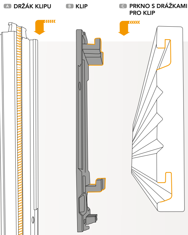
01 Upevnění «Držáku roštu» Techniclic®
