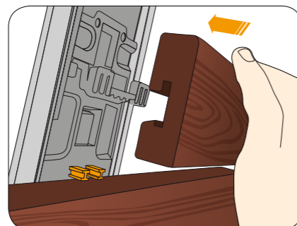
05 Montáž dalšího prkna
